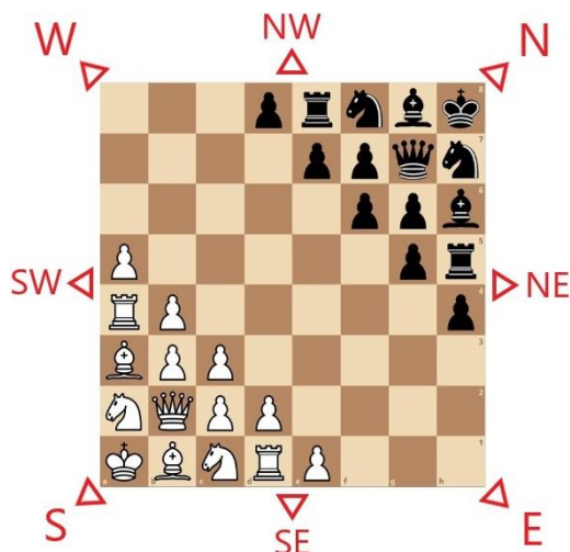
Rys. 2. Szachy diagonalne – orientacja szachownicy.
