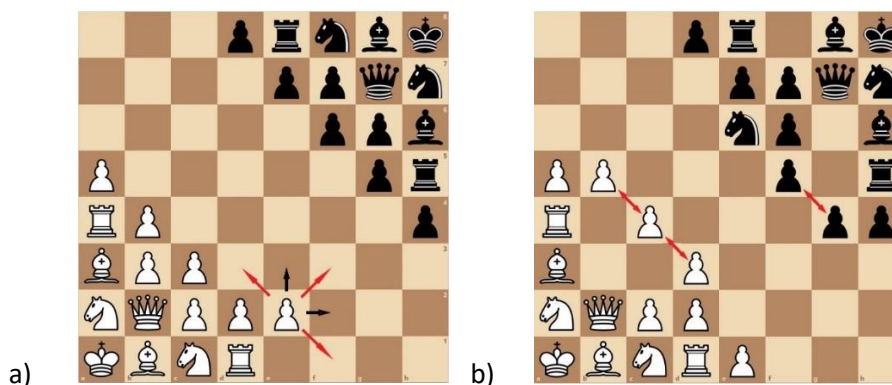
Rys. 5. Nowe możliwości pionów: a) ruchy i kierunki ataku; b) samoasekuracja.
