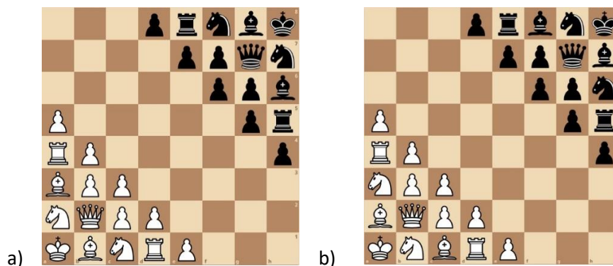
Rys. 4. Ustawienia początkowe: a) podstawowe; b) zwierciadlane w stosunku do osi N-S.
